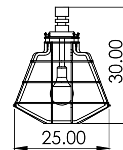
OCEAN MARINER MINI
